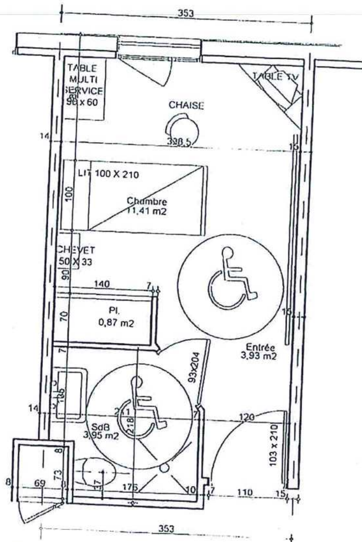
PLAN LOGEMENT TYPE échelle 1/50° Surface habitable : 20,16 m²
